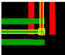
a) -shield_around_vias true (Default) Adds shields around vias.
