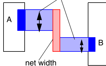
b) set_taper_width_nets -taper_style to_first_via
